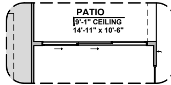
Stacking Door ILO Standard Door
